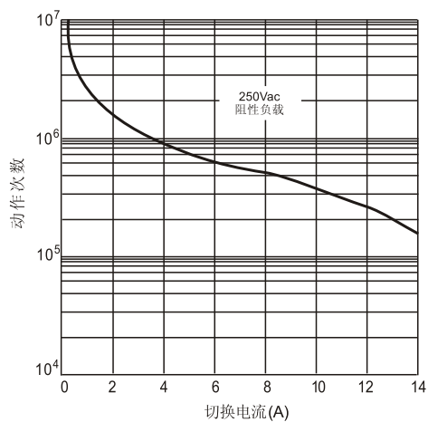
电气寿命
